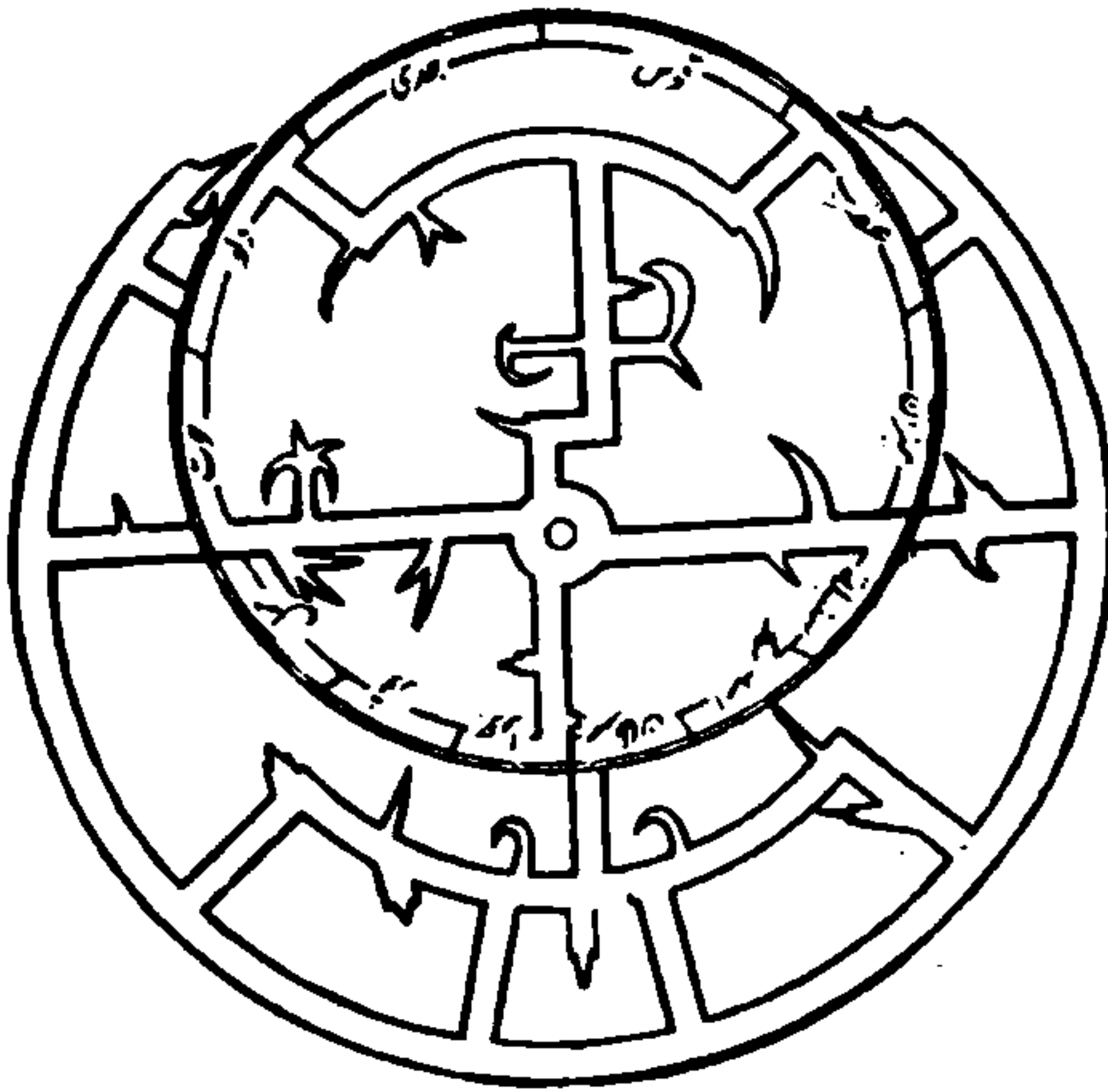
شکل ۲ - عنکبوتِ اسطرلاب
